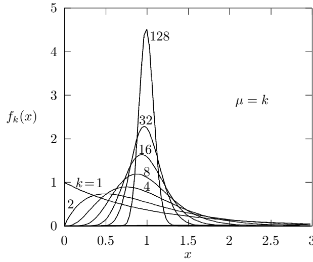
図 27: 平均 1 のアーラン分布の密度関数
