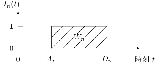
図 3: W_n と I_n(t) の関係
