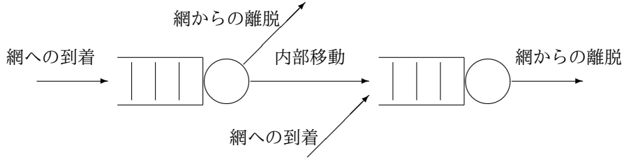
図 32: 待ち行列網
