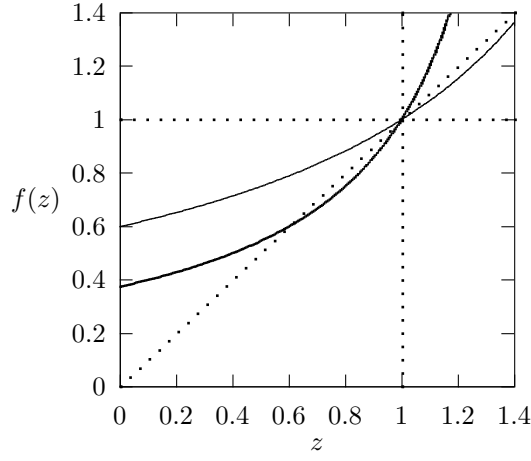
図 26: f(z) = G^*(\mu - \mu z) の挙動
