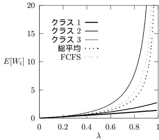
図 31: 非割込み優先規律における平均待ち時間 ( \lambda = 3\lambda^* )
