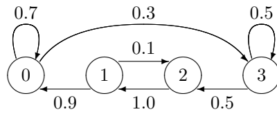
図 17: 状態遷移図の例 ( S = \{0, 1, 2, 3\} )
